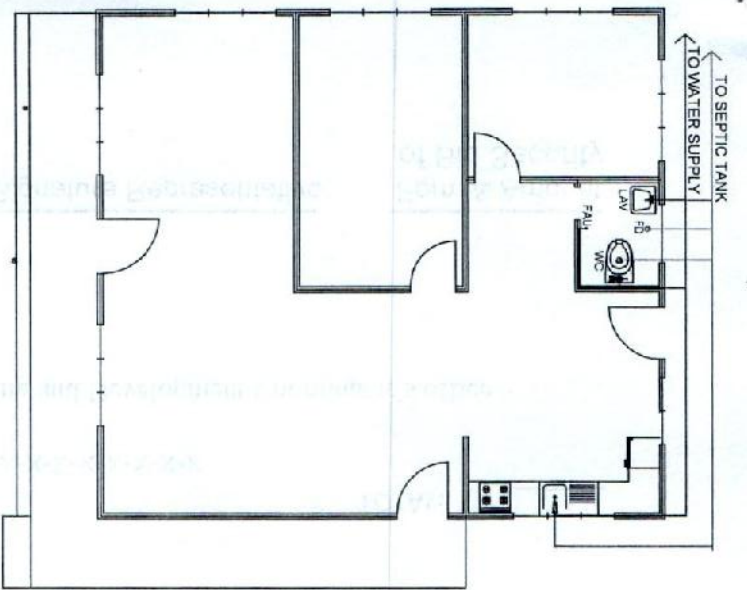
PLUMBING LAYOUT SCALE: 1:100
